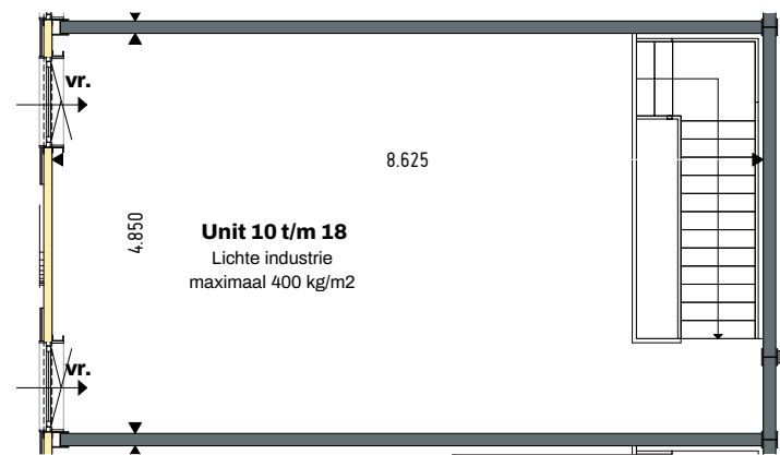
Verdieping 1:100
