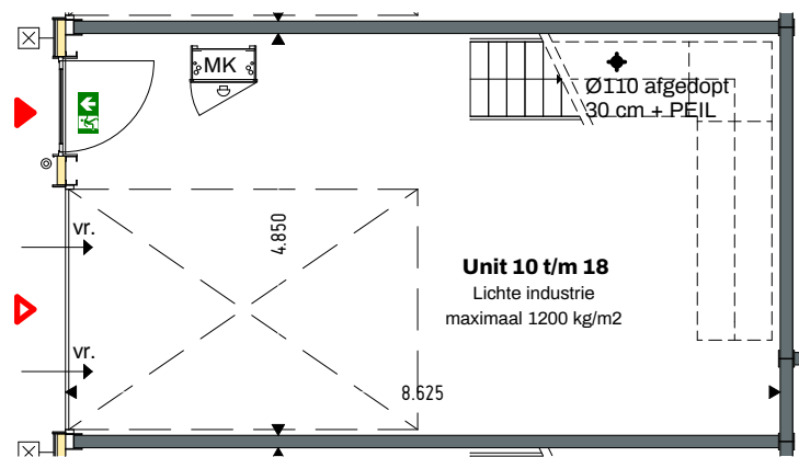
Begane grond 1:100
