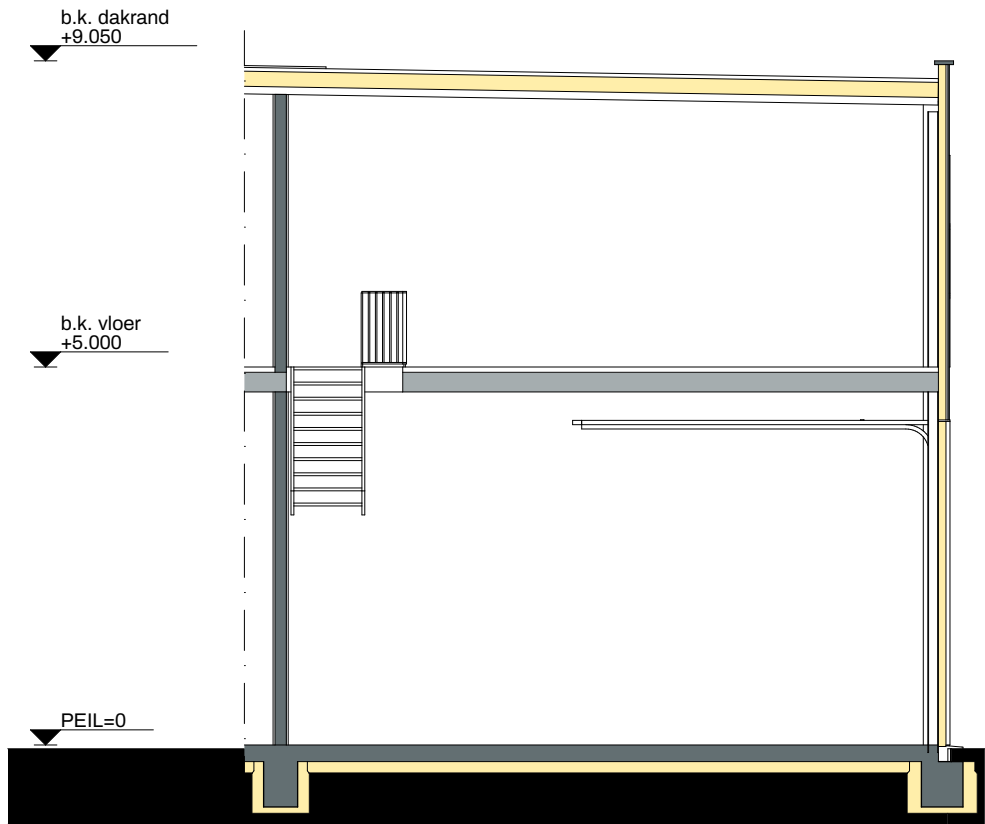
Doorsnede 1:100
