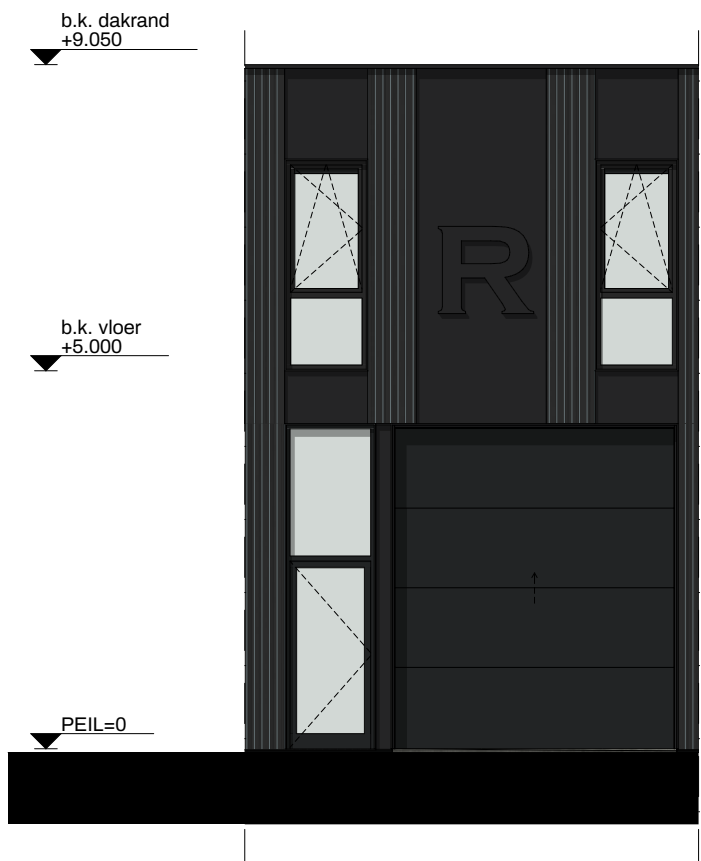
Voorgevel 1:100
